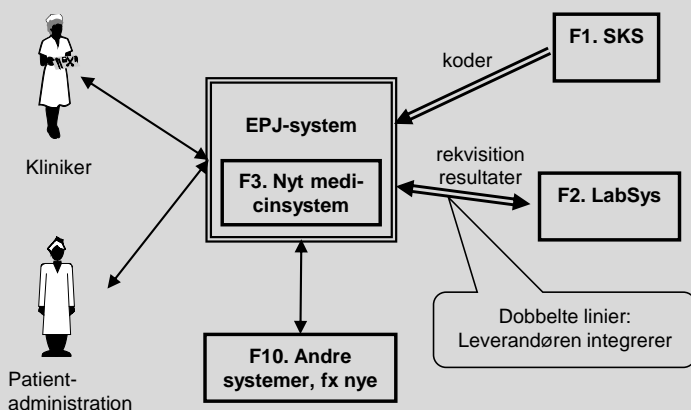
Figur 8. Kontekstdiagram
